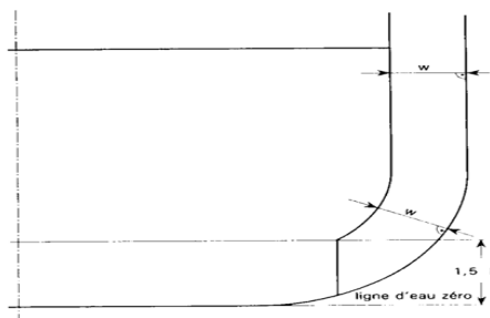
Figure 2 - Limites des citernes à cargaison aux fins du paragraphe 4
